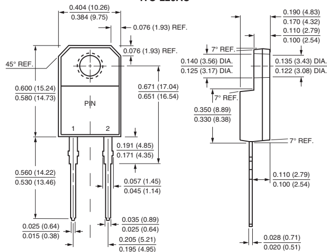
ITO-220AC
