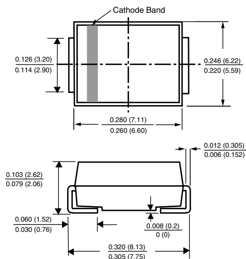
DO-214AB (SMCJ)
