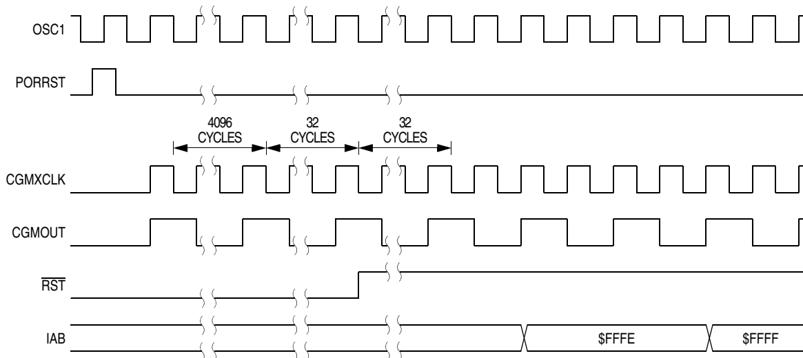
Figure 10-7. POR Recovery
