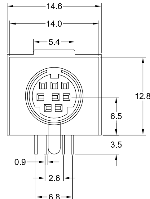
MDC-048 SHOWN
