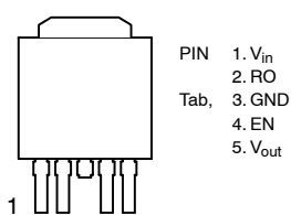
DPAK-5
