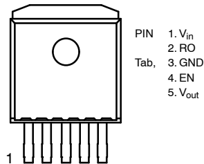
D 2 PAK-5
