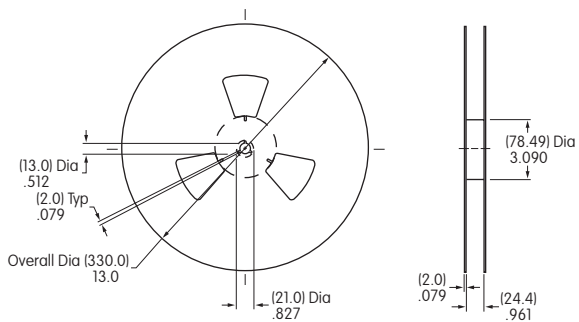
Reel Dimensions
