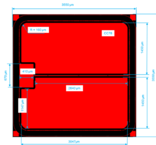
DIE OUTLINE
