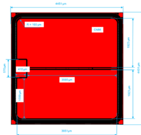
DIE OUTLINE
