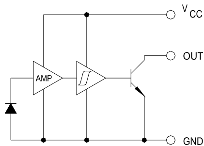
OPB686, OPB696 Buffered Open-Collector
