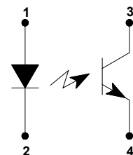
OPB860, OPB870, OPB880, OPB890
