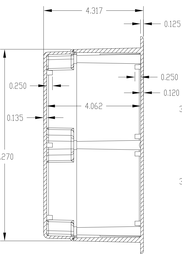
SECTION A-A
