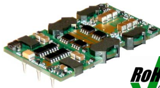
QD48T012033 Converter
