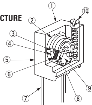
内部構造図
