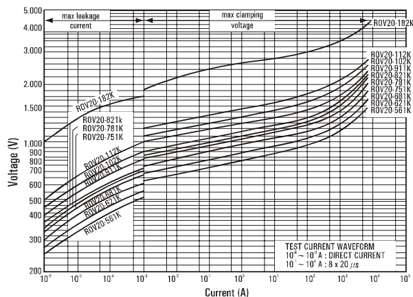
ROV20-561K – ROV20-182K
