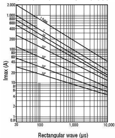
ROV20-220M – ROV20-680K
