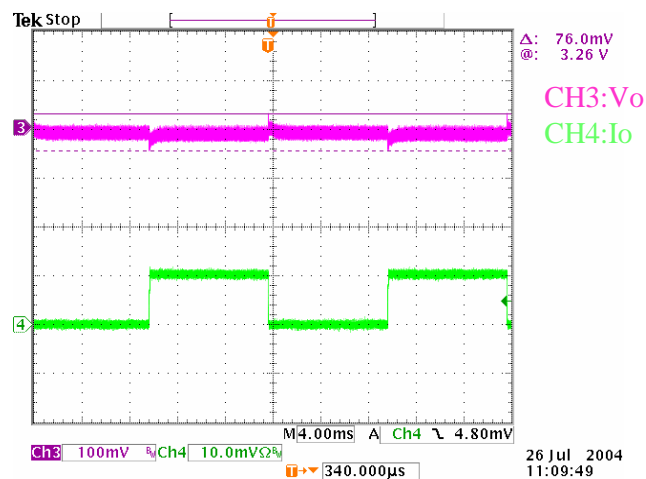
Transient response(0-5A).
