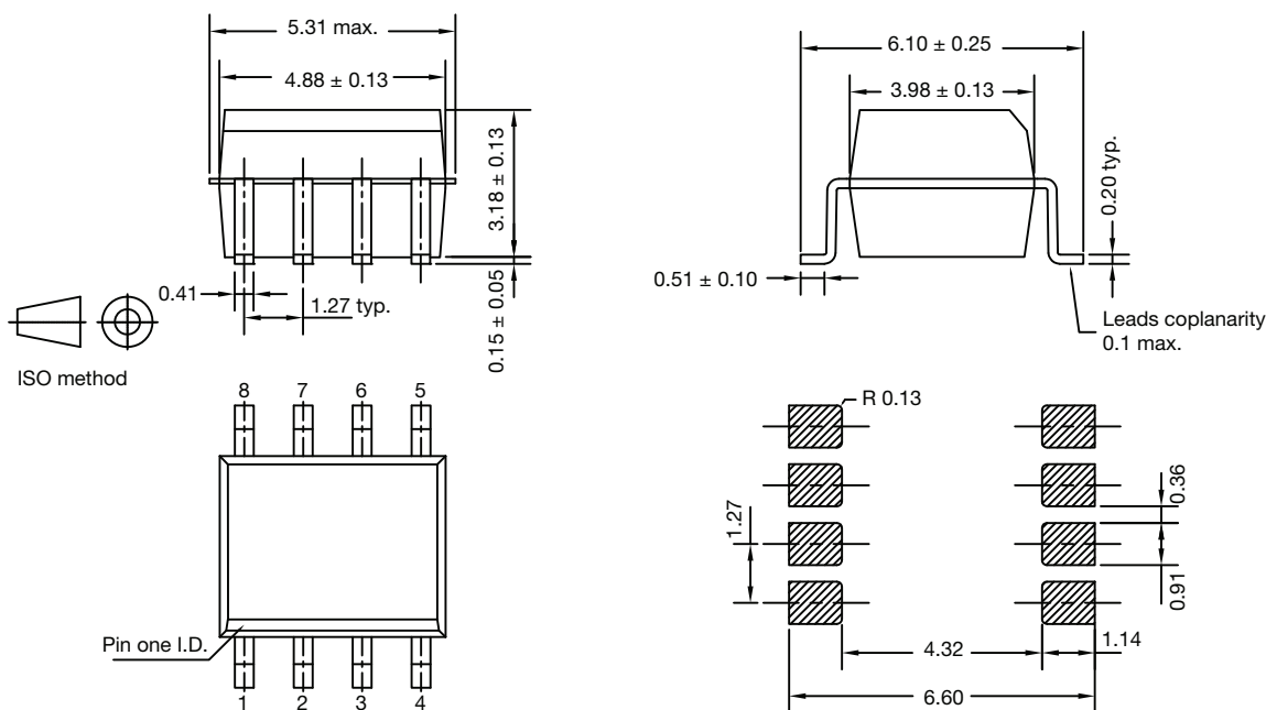
Fig. 21 - Package Dimensions
