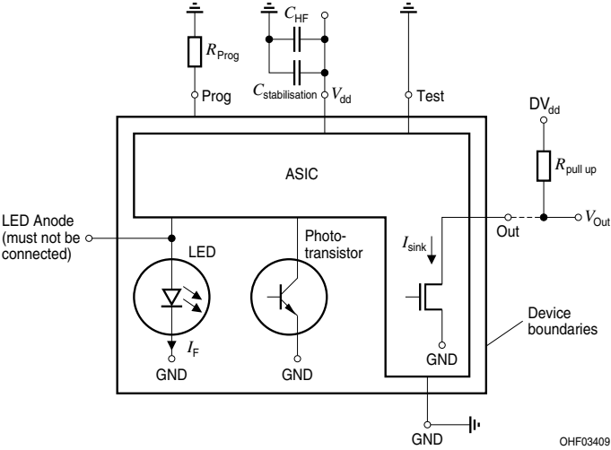
Blockschaltbild 4) Seite 16
