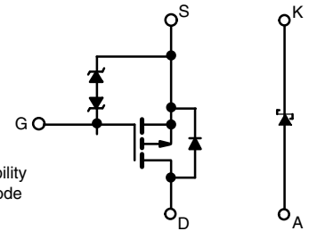
P-Channel MOSFET
