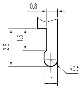
K DETAIL 2 : 1
