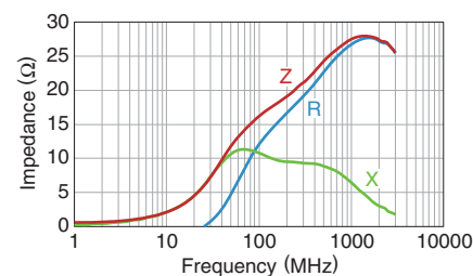
MMZ2012Y150BT000
