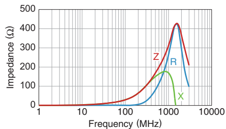
MMZ0603D800CT000
