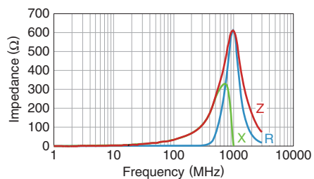
MMZ1005F330CT000
