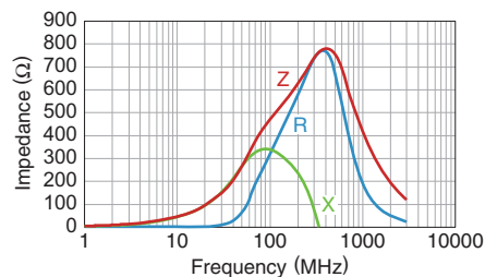
MMZ0603D470CT000
