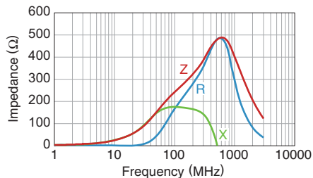
MMZ0603Y241CT000
