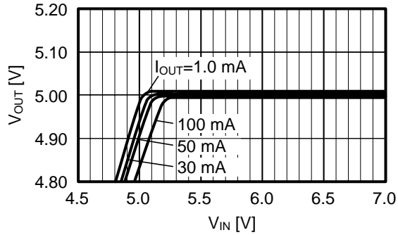
S-L2980A50 ( T_a=25^\circ\text{C} )
