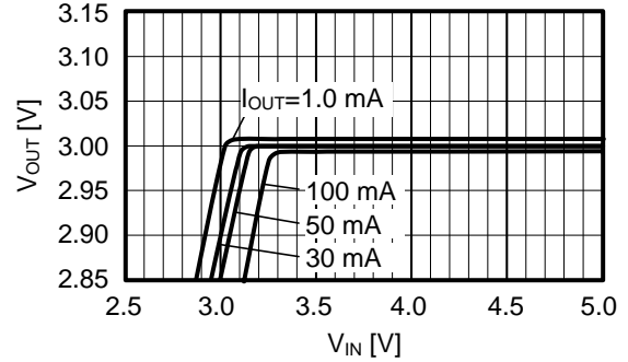
S-L2980A30 ( T_a=25^\circ\text{C} )
