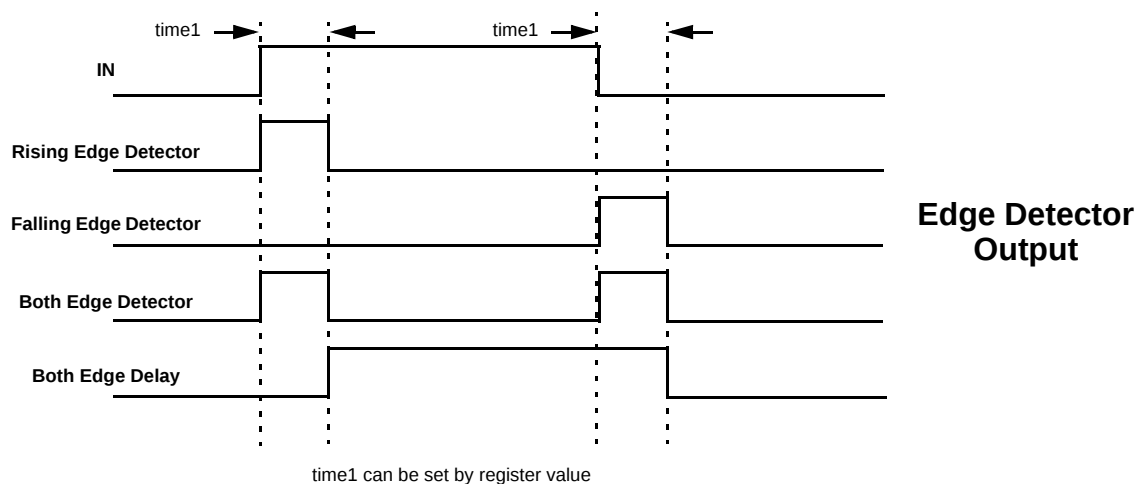
Figure 15. Edge Detector Output
