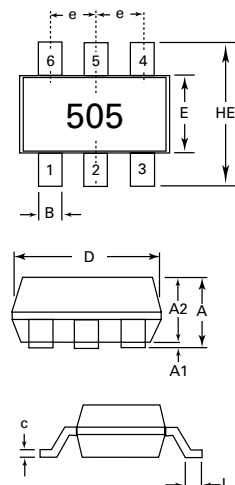
SP0505BAJTG - SC70-6
