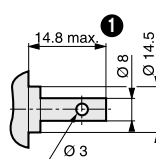
Shaft 79 261 309
