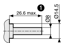
Shaft 79 261 300
