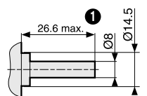
Shaft 79 261 300
